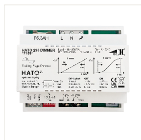
HATO 230 DIMMER (Variation de phase)
